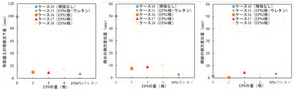
i : 背面盛土の残留沈下量 (V1) ii : 橋台の側方変位量 (H1) iii : 橋脚の側方変位量 (H2) 図-23 EPSの量と背面盛土の残留沈下量、及び橋台・橋脚の側方変位量の関係
