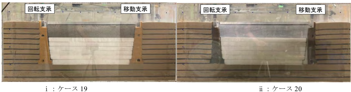
図-28 5回加振終了時の土槽側面写真
